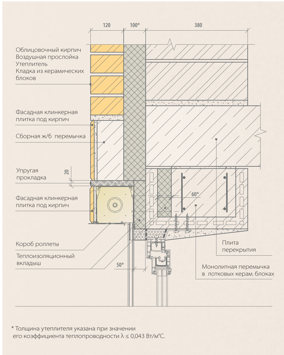
Температурное поле
