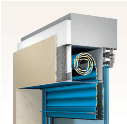
Встроенный короб SB-1/m Типоразмеры: 137...205 мм
